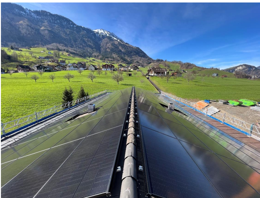
Photovoltaikanlage auf dem Dach des Alters- und Pflegeheims Nidwalden in Stans
